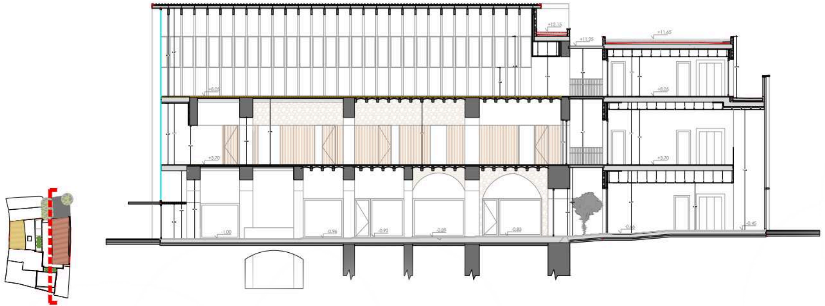
Secció Transversal T1
